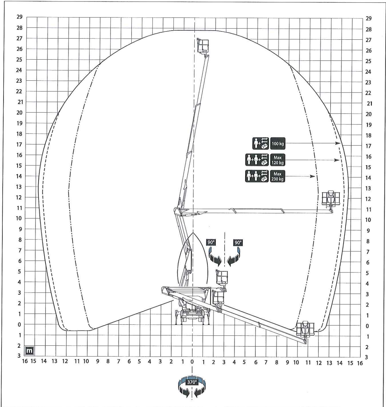
Diagramma area di lavoro con bracci stab. estesi
